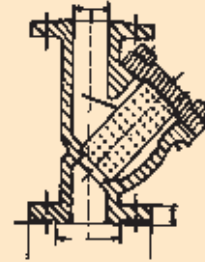
Y TYPE STRAINER
